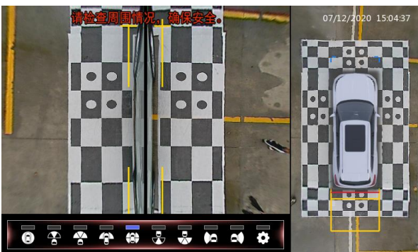
图6-7: 2D过窄道模式
